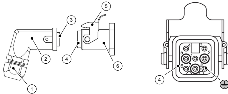
Fig. 11: HAN connector
